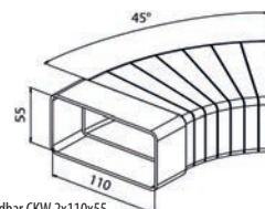
Állítható könyök idom (45°) / Flachkanal-Bogen, abscheidbar CKW 2x110x55
