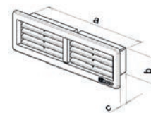
Szellőzőrács lapos légszatórnához / Lüftungsgitter zum Belüftungssystem VM 110x55 biela
