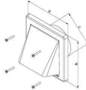
GK - Gravitációs visszacsapó szelep / Gravitationsklappen
